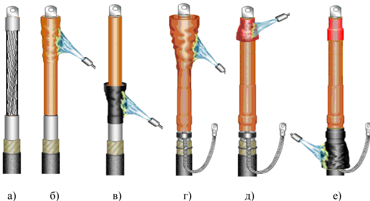
Рис. 3.8. Монтаж концевой термоусаживаемой муфты:
