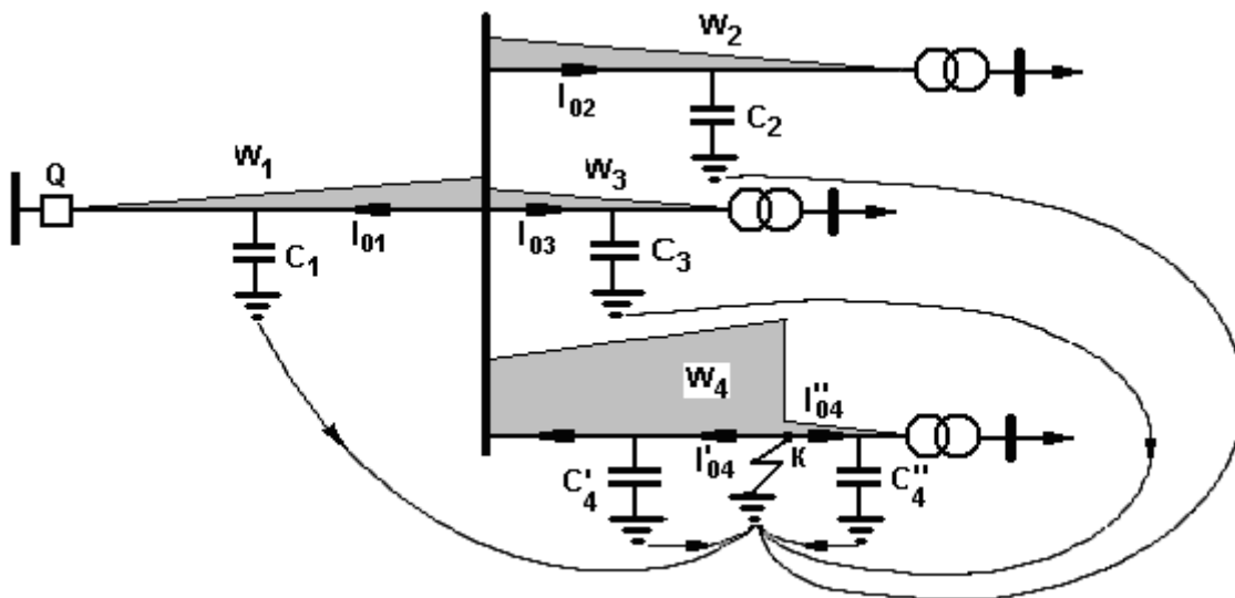
Рис. 7.3. Схема сети и эюры показаний переносного прибора в различных ее участках
