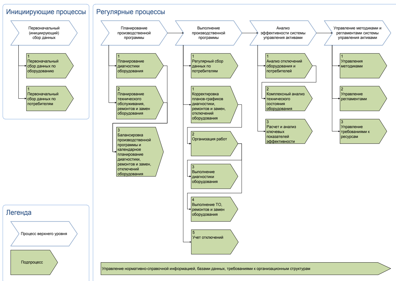
Рис. 3. Схема процесса управления производственными активами верхнего уровня
