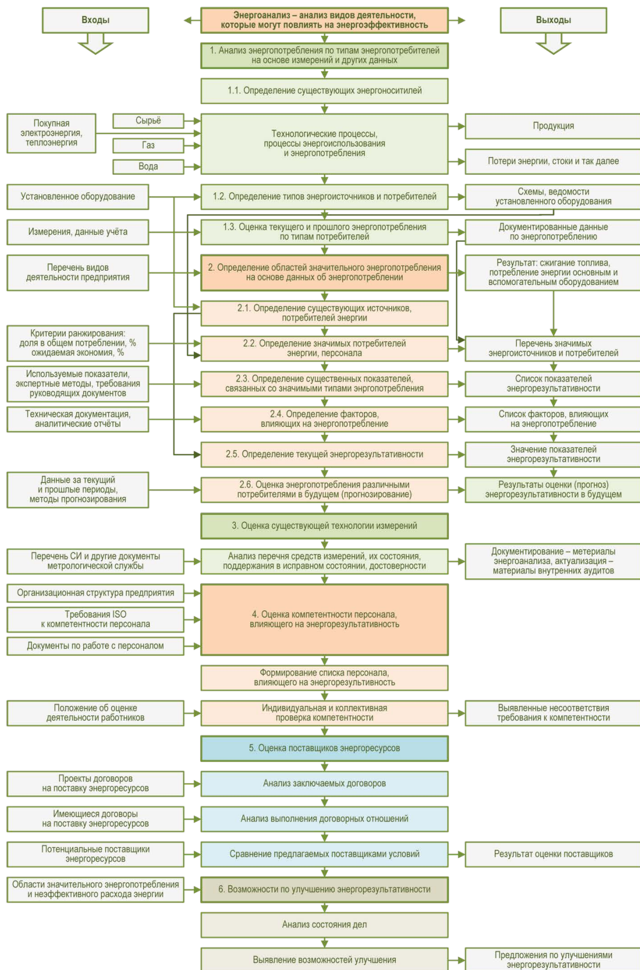
Рисунок 17 – Схема энергоанализа нефтеперерабатывающего завода
