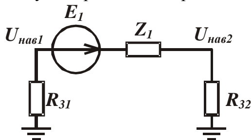
Рисунок 4 Схема замещения для расчета наведенных напряжений на участке ВЛ, заземленной в двух точках
