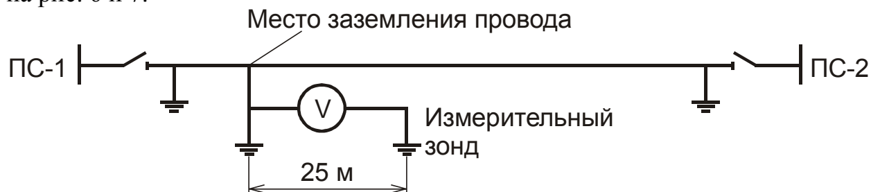
Рисунок 6 Принципиальная схема измерения наведенного напряжения
