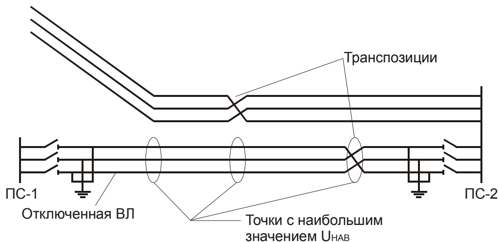
Рисунок 5 Места наибольших значений наведенного напряжения на проводах отключенной ВЛ
