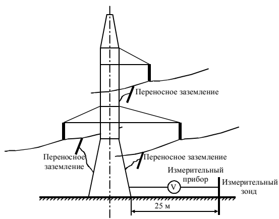
Металлическая или железобетонная опора
