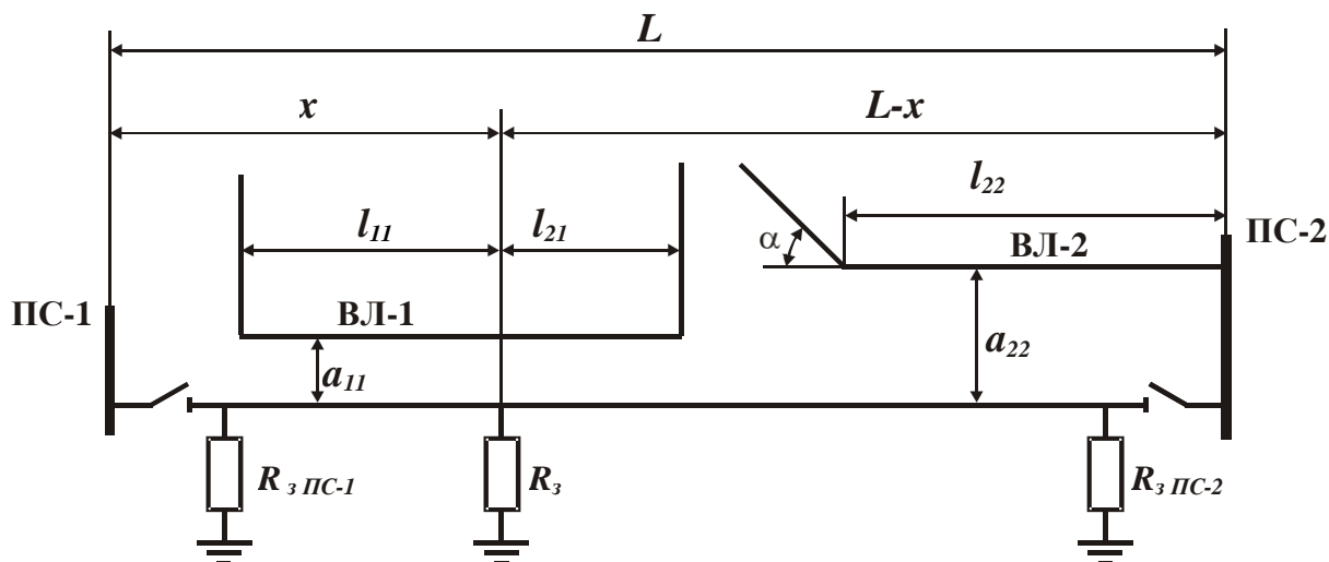
Рисунок 3 Топографическая схема сети при наличии влияющей линии, наводящей ЭДС в левом и правом контуре
