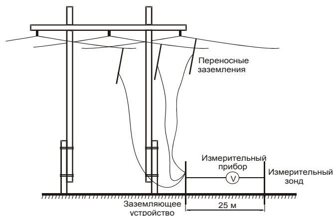
Деревянная опора (без заземляющего спуска)
