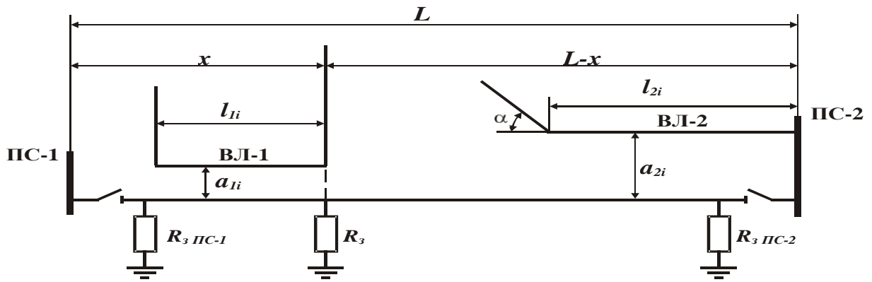
Рисунок 2 Топографическая схема сети
