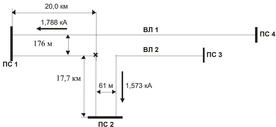
Рисунок П1 - Схема сети 500 кВ
