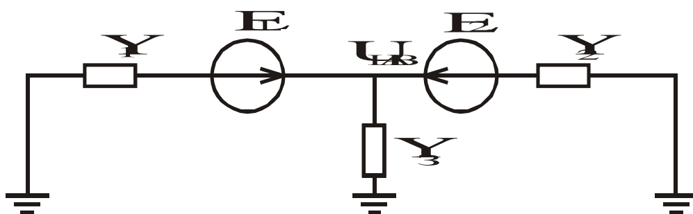
Рисунок 1 Схема замещения для расчета значения наведенного напряжения на отключенной ВЛ
