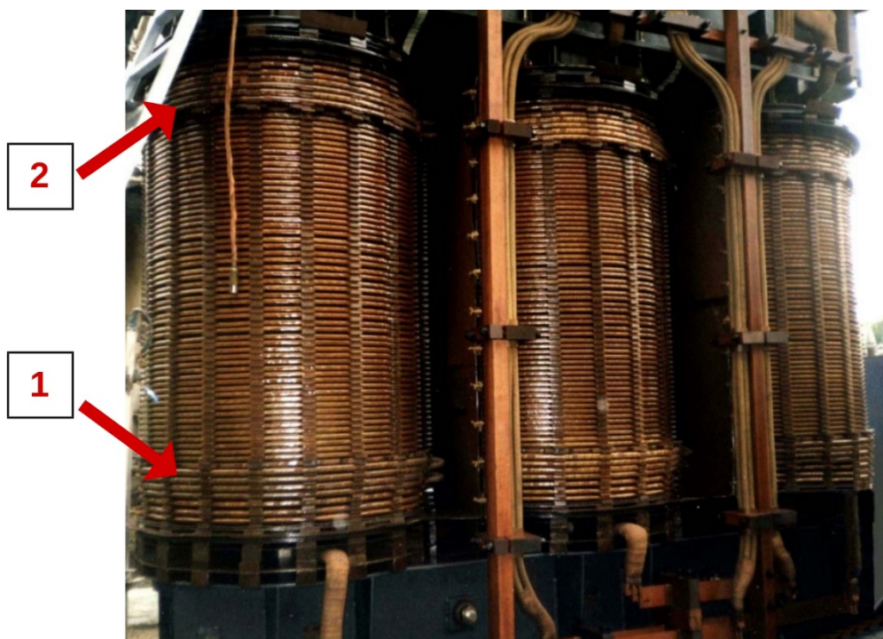
Рисунок 2 – Пример конструкции с вводом линейного напряжения с верхнего и нижнего торца обмотки ВН
