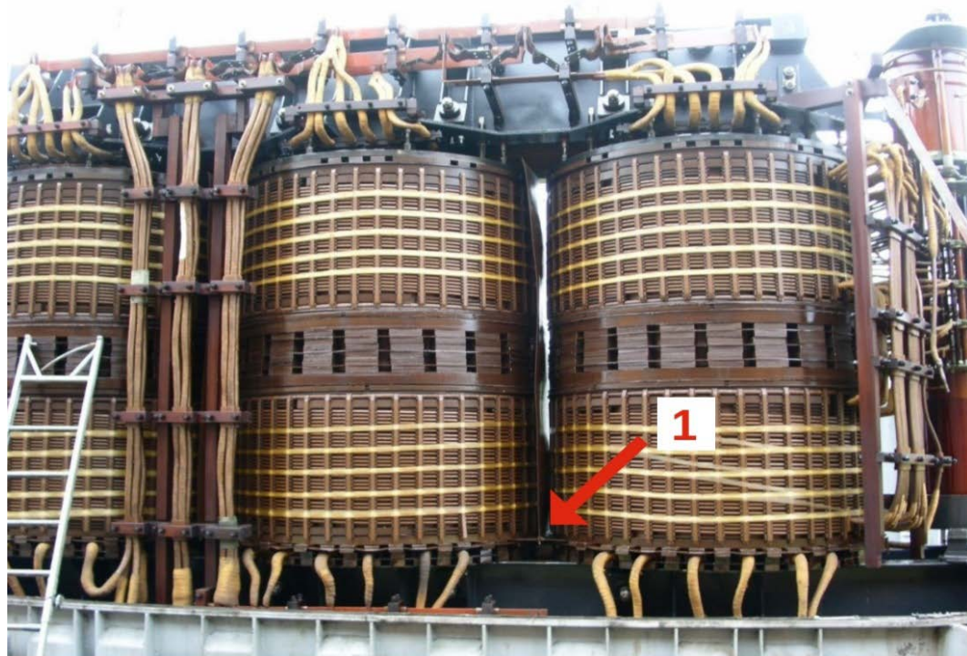
Рисунок 10 – Пример конструкции с наружной РО класса 35 кВ
