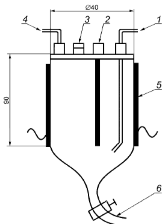
Рисунок В-5 – Стеклоанный сосуд испарителя с нагревателем
