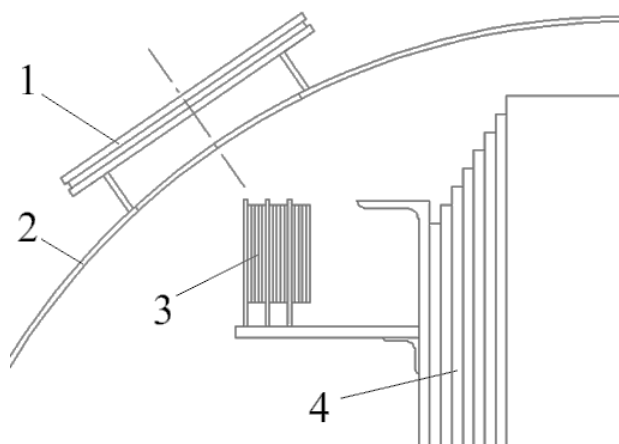
Рисунок 1 – Эскиз расположения макета изоляции в баке колокольного типа: 1 – люк; 2 – бак трансформатора; 3 – макет изоляции; 4 – магнитопровод.
