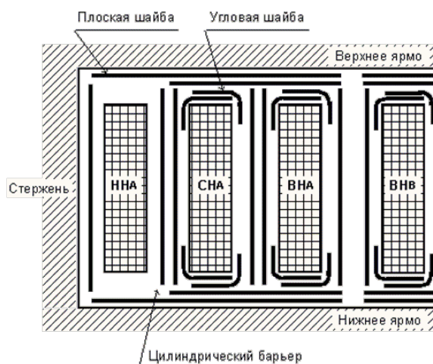
Рисунок А1 – Общий вид главной изоляции обмоток трансформаторов
