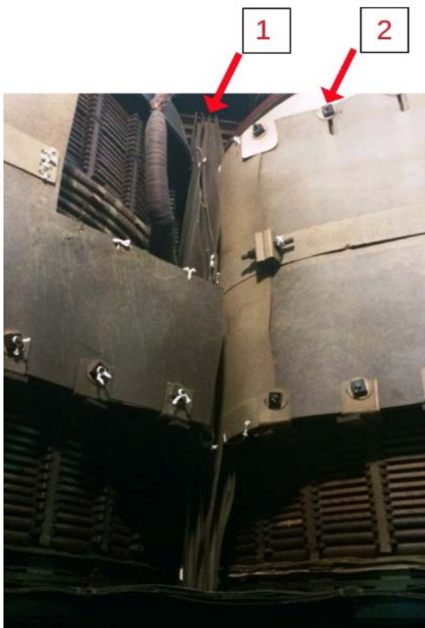
Рисунок 5 – Пример конструкции с многослойной межфазной перегородкой и зоны отбора образцов
