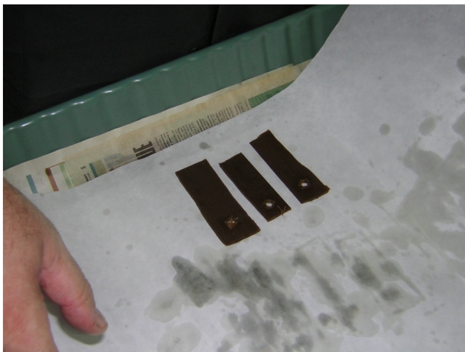
Рисунок Б-8 – Протирка изоляции фильтровальной бумагой
