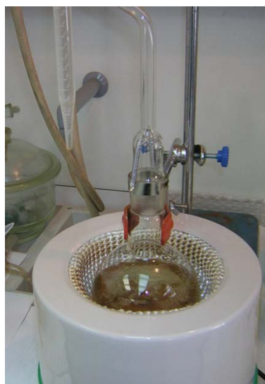
Рисунок Б-14 – Колба с образцами в колбонагревателе после удаления стеклоткани
