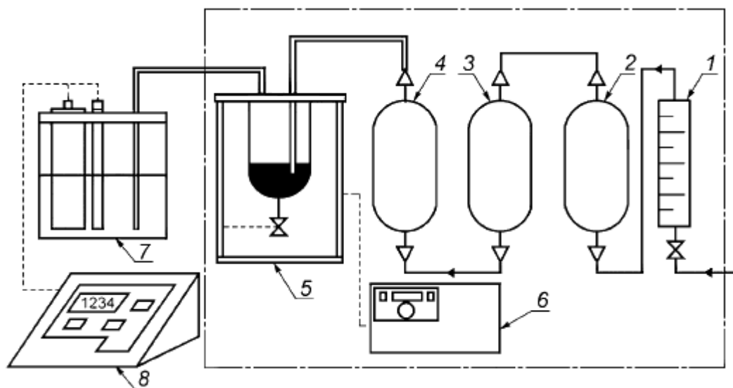
Рисунок В-4. Блок-схема автоматического титратора и блока для выпаривания.
