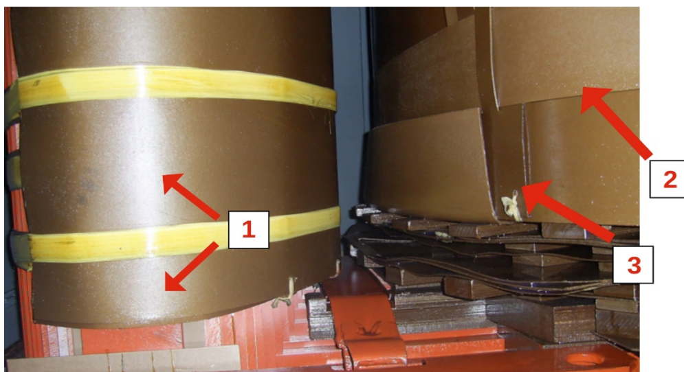
Рисунок 11 – Пример конструкции с барьером по всей высоте обмотки ВН, барьером на боковом ярме и зоны отбора образцов
