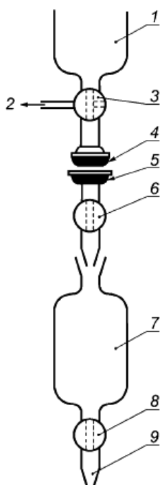
Рисунок В-3 – Контейнер для метанола и трубка для экстрагирования:
