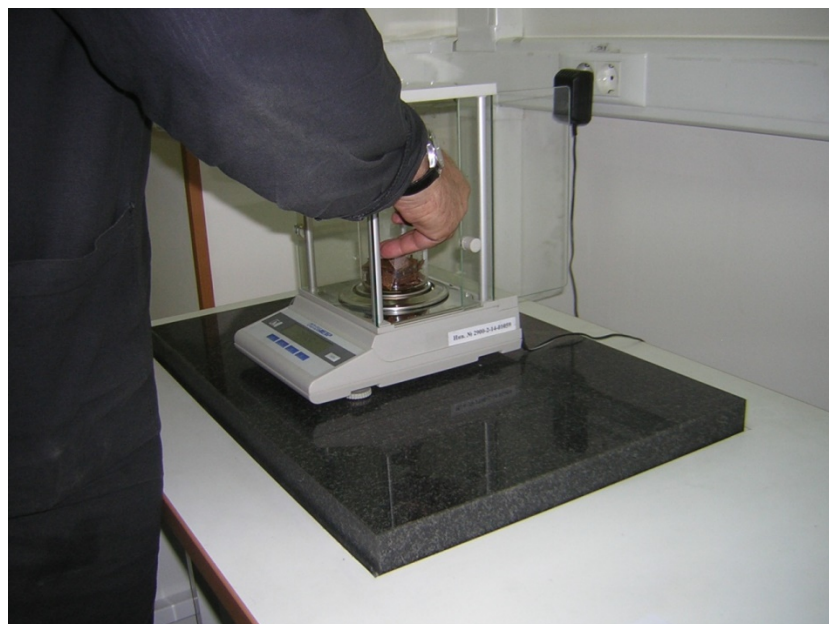
Рисунок Б-11 – Взвешивание навески образца изоляции
