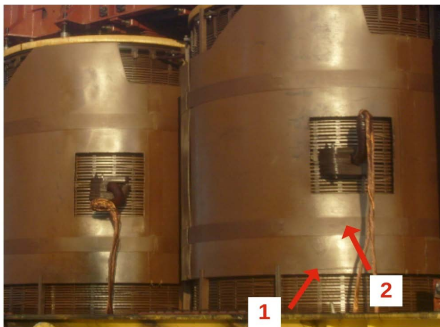
Рисунок 8 – Пример конструкции с облегающими обмотки ВН барьерами и зоны отбора образцов
