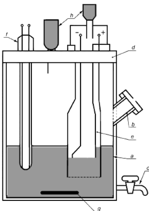
Рисунок В-2. Подходящий сосуд для титрования в сборе.
