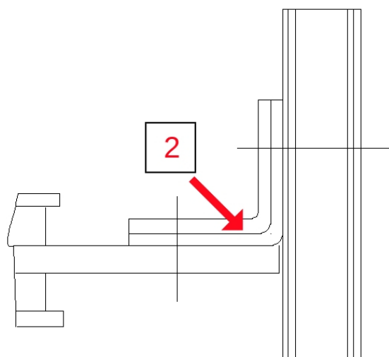
Рисунок 7 – Эскиз крепления укороченного наружного барьера и зона отбора образцов
