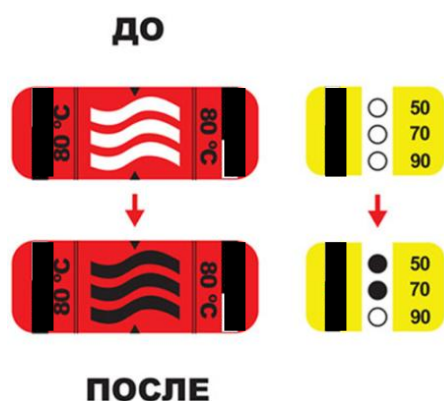
Рисунок 13. Примеры термоиндикаторных наклеек различных производителей
