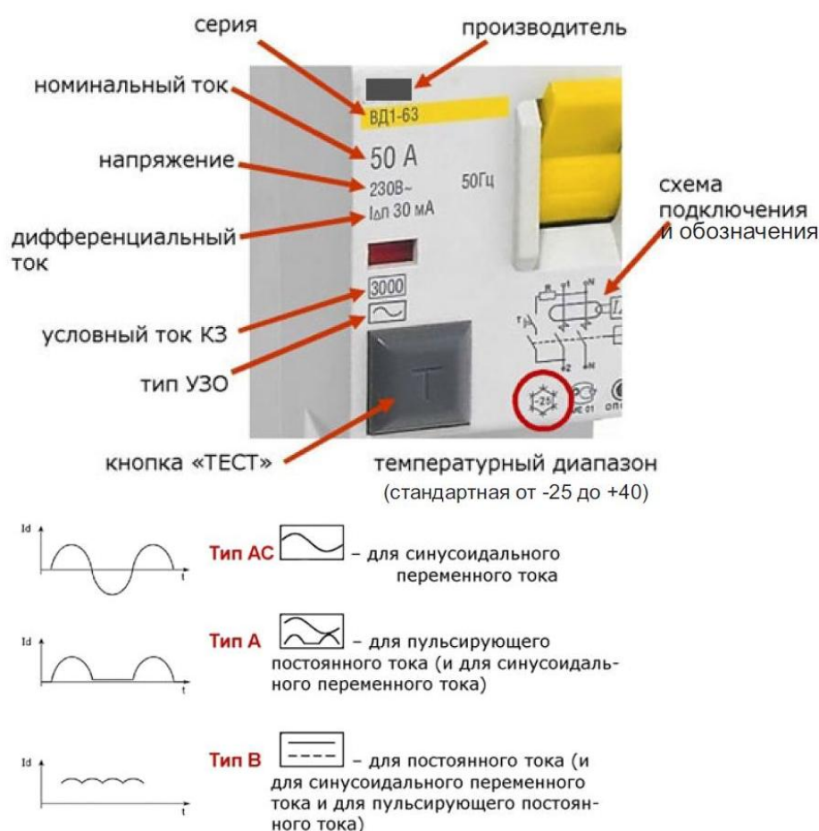
Рисунок 5. Маркировка УДТ
